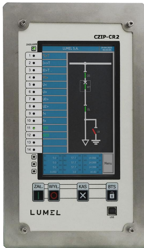
Rys. 11.1. Widok płyty czołowej zespołu CZIP-CR2.
